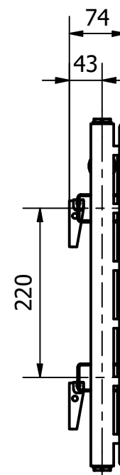
LUXRAD Niagara pozioma z wkładką termostaticzną 445x1500
