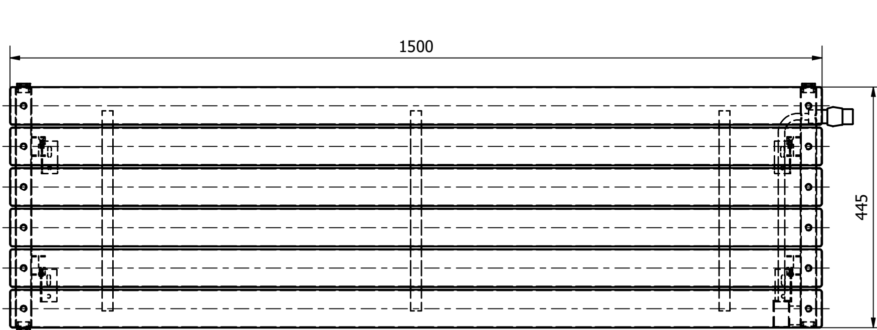
LUXRAD Niagara pozioma z wkładką termostaticzną 445x1500
